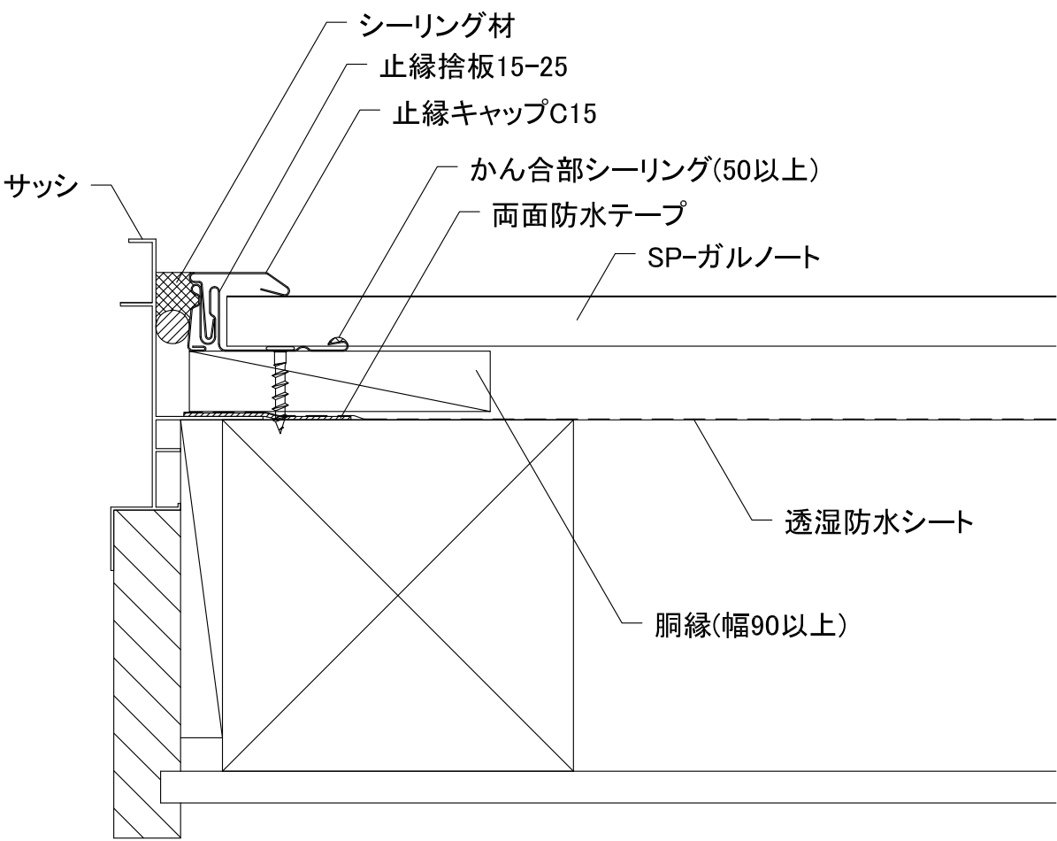
開口部左右
