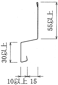
断面詳細図
