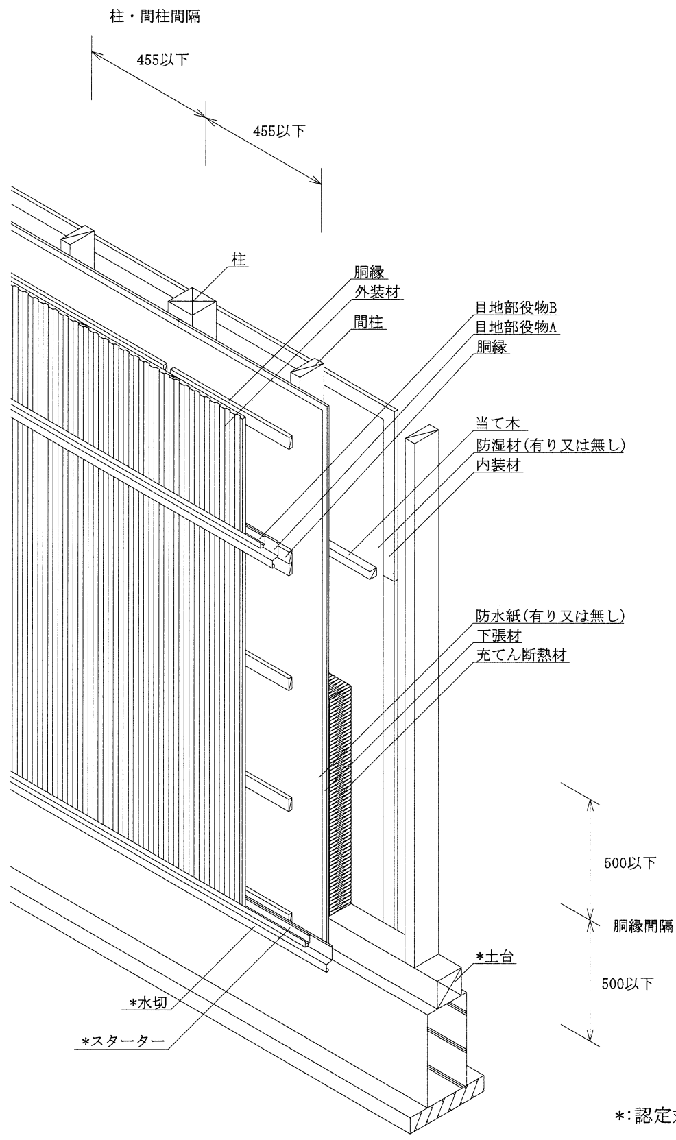
透視図 (別添 - 15)
