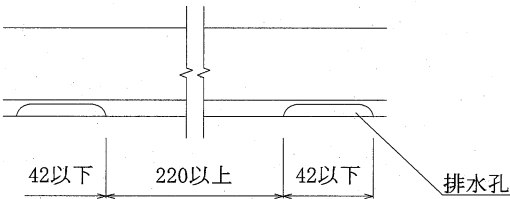
背面図
