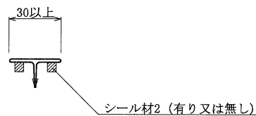
キャップA (ピース材)
