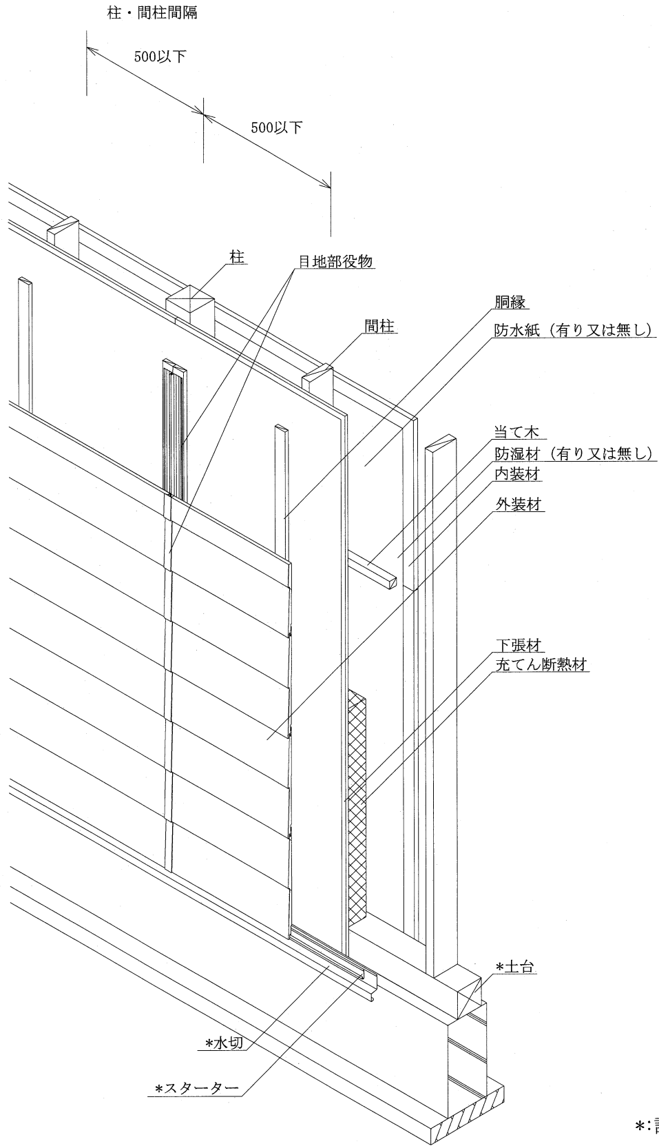
透視図 (別添 - 14)
