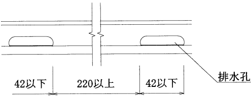
背面図
