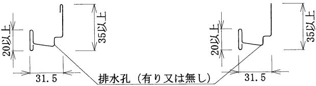
断面詳細図
