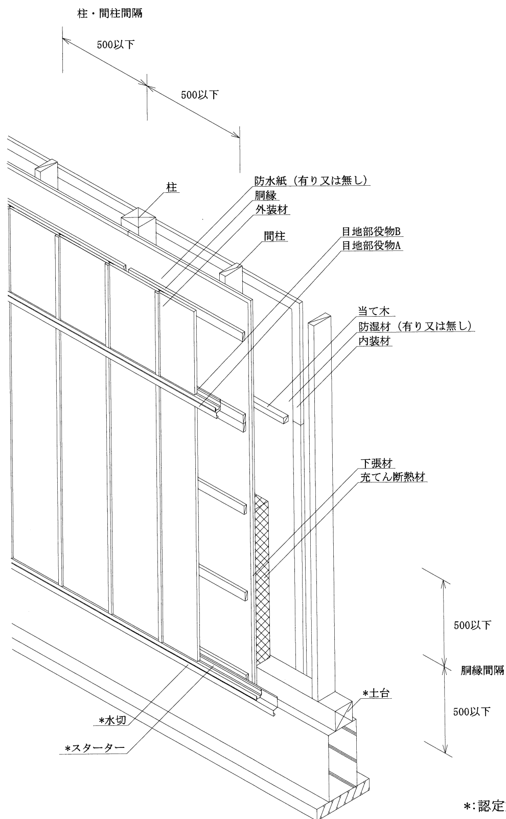
透視図 (別添-14)
