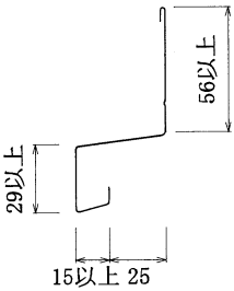
断面詳細図
